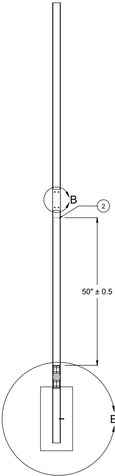
SECTION A-A
